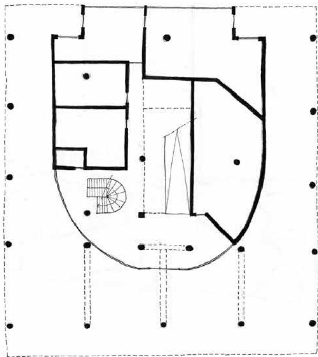
Plan du rez-de-chaussée
